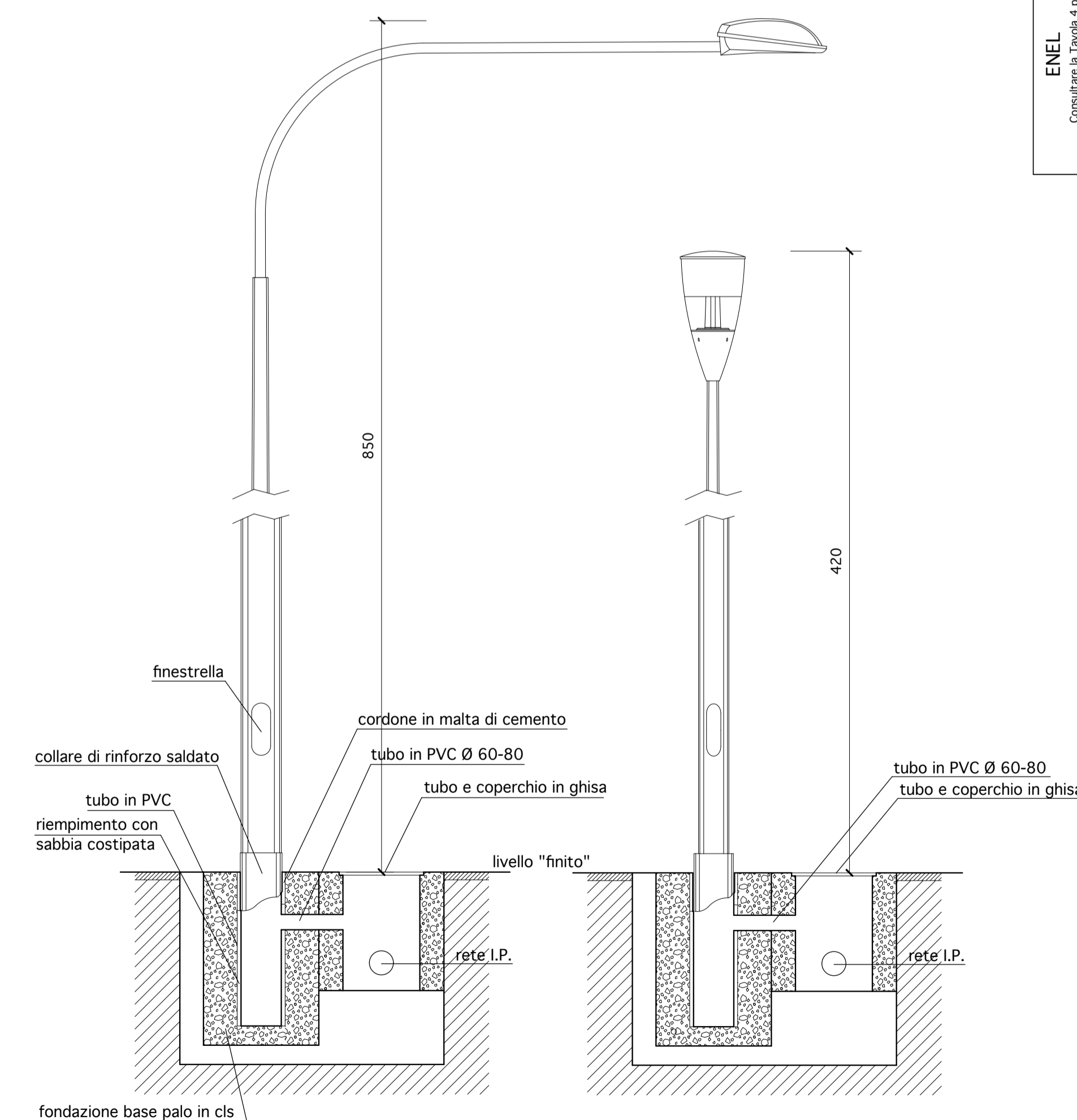
PARTICOLARE DELLA FONDAZIONE DEI PALI DI PUBBLICA ILLUMINAZIONE Scala 1:25
