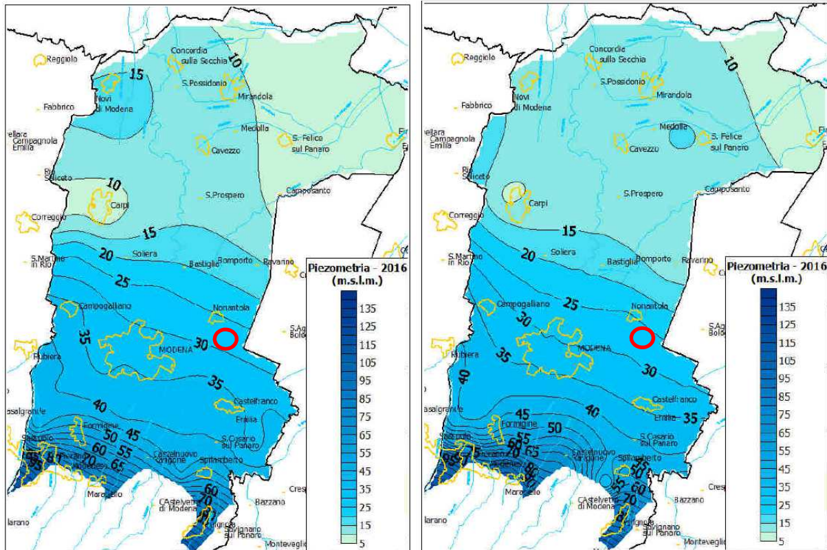
Figura 10 – Andamenti piezometrici nei corpi idrici liberi e confinati superiori (a sinistra) e nei corpi idrici liberi e confinati inferiori (a destra). Fonte: Report Arpae 2016 “La qualità delle acque sotterranee in Provincia di Modena” (2018).
