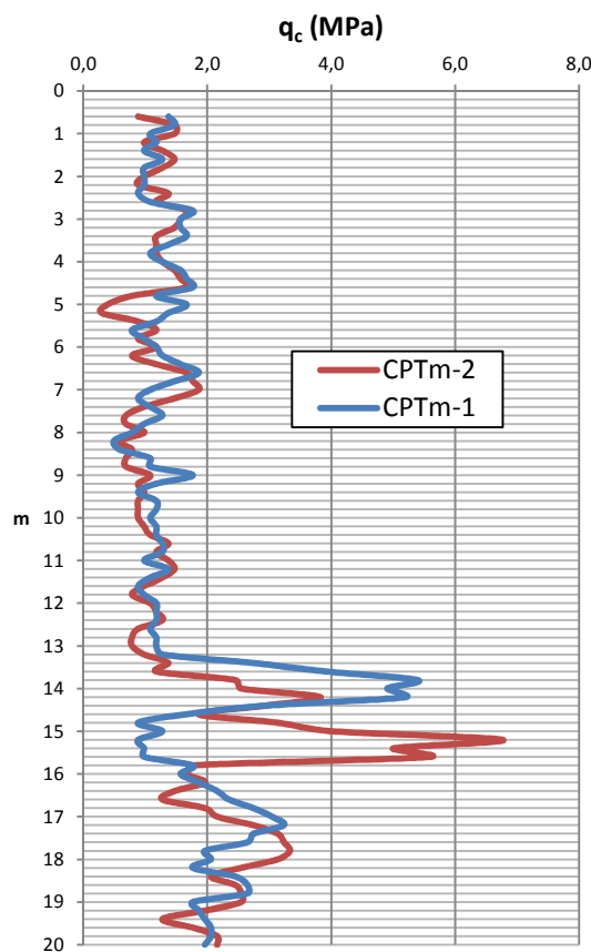
Figura 12 – Confronto dei profili di R_p con la profondità delle due verticali penetrometriche.
